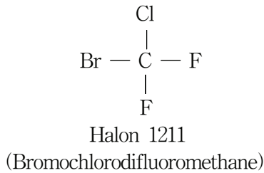
[그림 2] 대표적인 할로겐화합물 소화약제의 구조식
