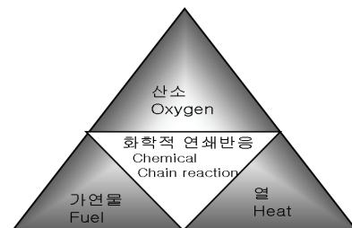
[연소의 4요소]
