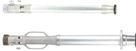
[직사형 폼 노즐]
