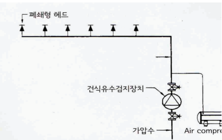
건식(Dry pipe system)
