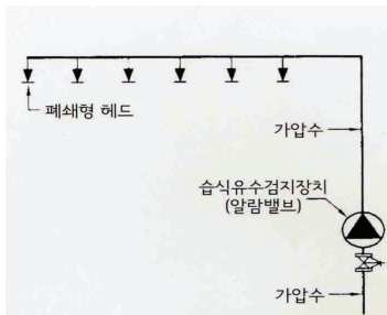
습식(Wet pipe system)
