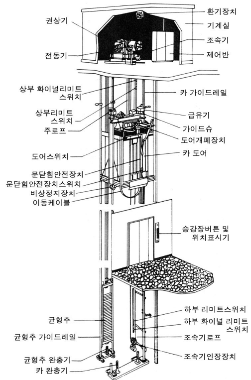
(그림 5-99) 엘리베이터의 구조
