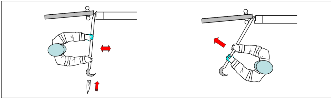
(그림 6-20) 지렛대 활용 작업(1)
