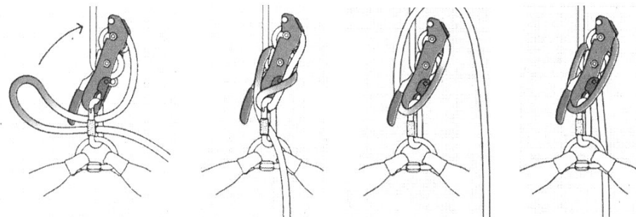
(그림 3-80) 스톱하강기 고정법
