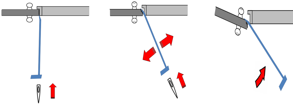
(그림 6-24) 지렛대 활용 작업(3)
