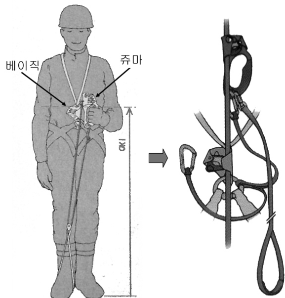
(그림 3-83) 슬링의 길이를 적절히 조정한다.
