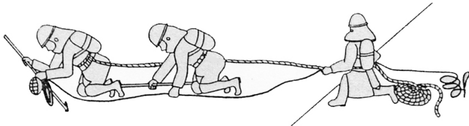
(그림 4-40) 농연 속에서는 자세를 낮추고 진입한다. 선 진입자에게 유도로프를 결착하여 후진입자가 이를 잡고 진입할 수 있도록 한다.
