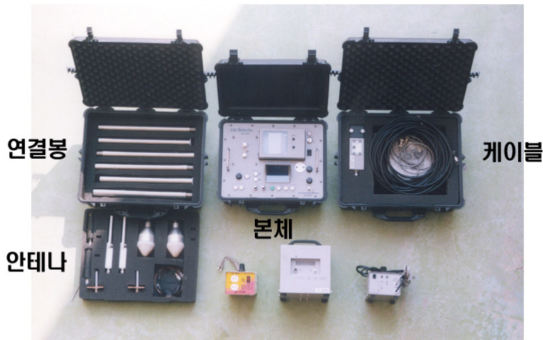
(그림 2-20) 매몰자전파탐지기
