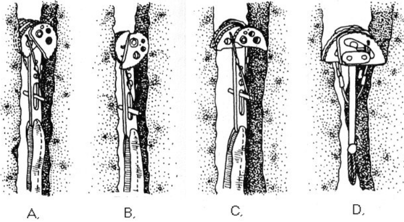
(그림 5-117) 프랜드(캠) 설치하기
