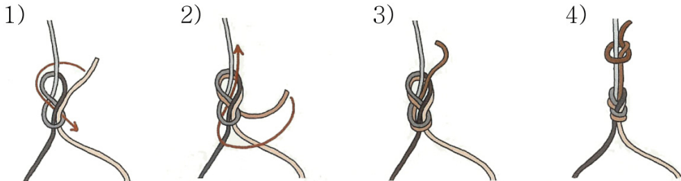
(그림 3-16) 움매듭은 8자연결매듭에 바짝 붙이는 것이 좋다.
