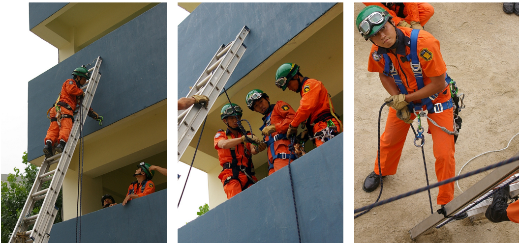
(그림 4-20) 가로대 위로 로프를 빼 내어 안전벨트에 걸착한다.
