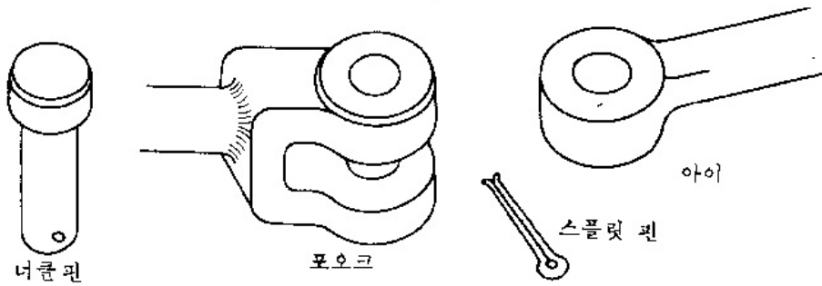
(그림 5-12) 링크로 연결된 부분은 먼저 스플릿 핀을 제거하고 너클핀을 뺀다.
