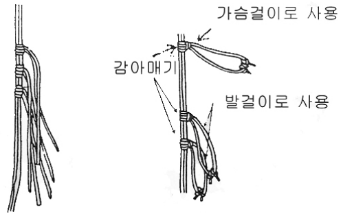
(그림 3-90) 감아매기 등반 로프 만들기
