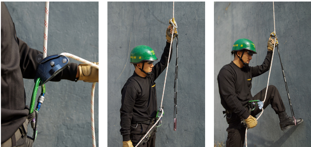
(그림 3-86) 그리그리와 주마에 현수로프를 삽입한다. 슬링의 고리에 발을 넣고 힘차게 일어선다.
