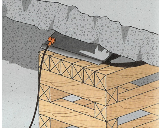
(그림 2-9) 받침목을 이용한다.
