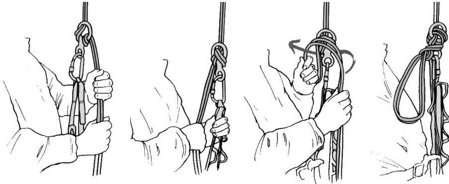
(그림 3-78) 8자 하강기를 완전히 고정하는 방법
