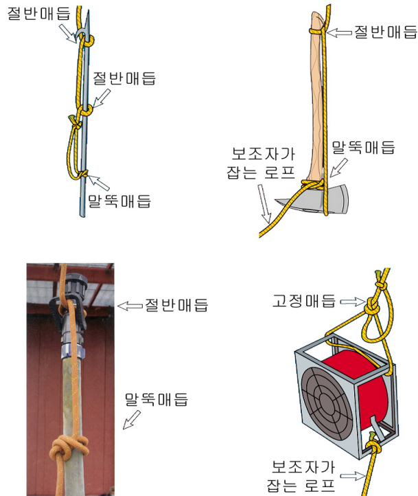
(그림 3-29) 여러가지 기구 묶기
