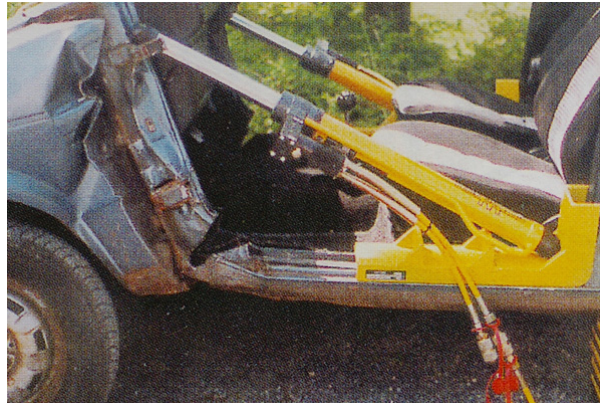
(그림 2-13) 유압램을 확장시켜 차체를 밀어낼 수 있다.
