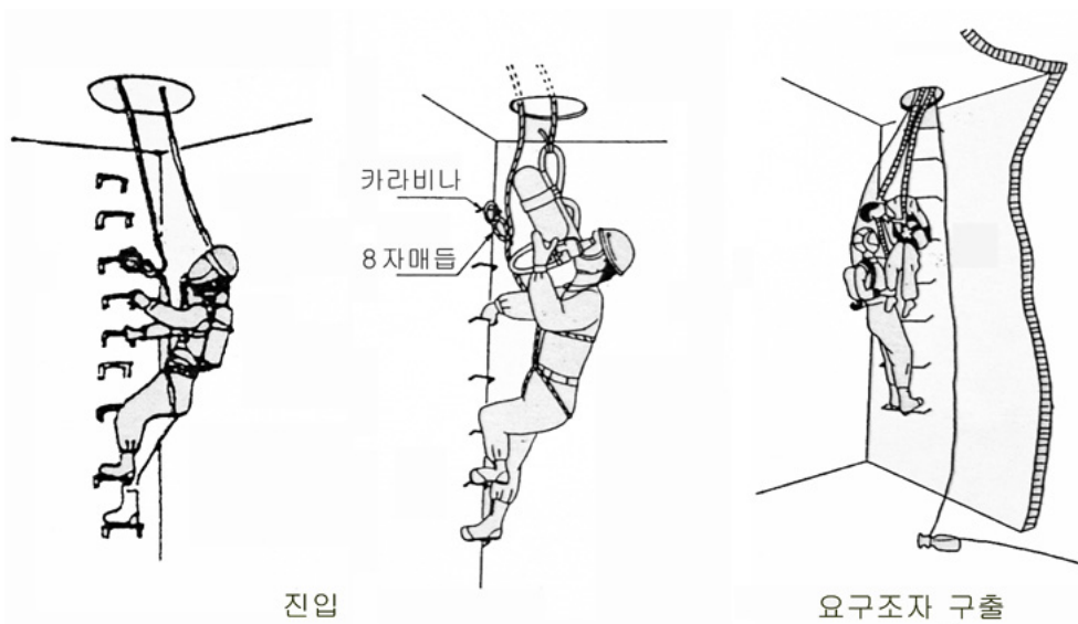
(그림 4-38) 폐쇄공간에서 요구조자 구출방법
