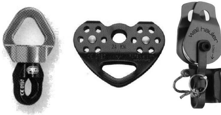
(그림 2-30) SWIVEL
