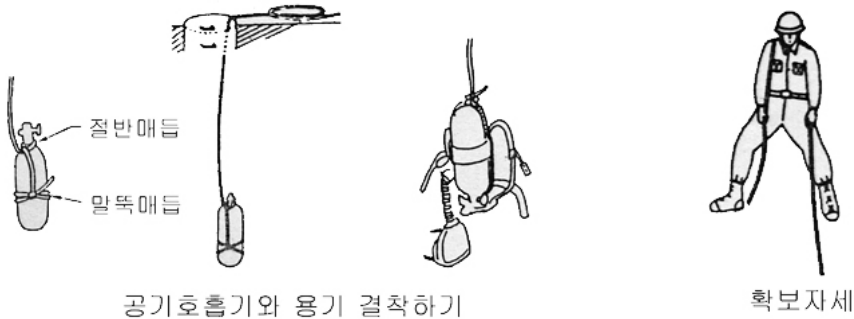
(그림 4-37) 폐쇄공간 진입법
