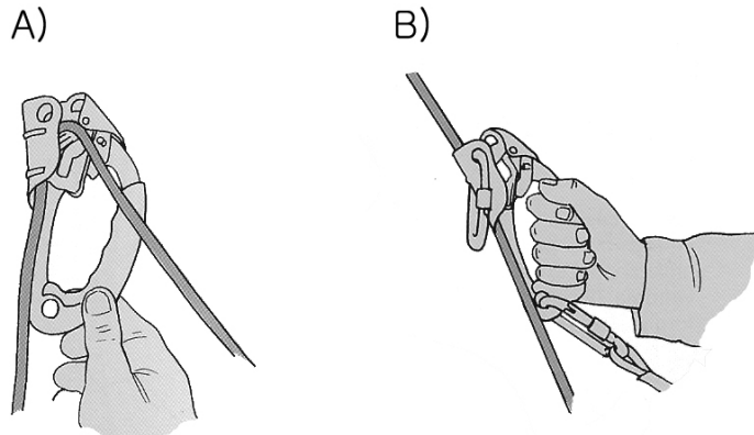
(그림 3-85) 로프가 이탈하지 않도록 카라비나를 끼워둔다.
