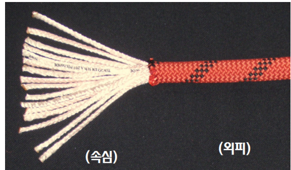
(그림 2-1) 쾨먼틀 로프의 구조
