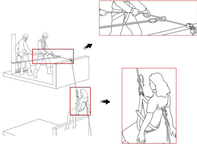
(그림 4-14) 요구조자 수직 하강시키기
