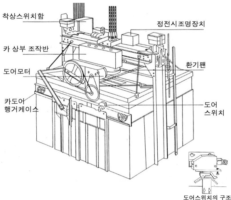
(그림 5-100) 카 상부의 구조
