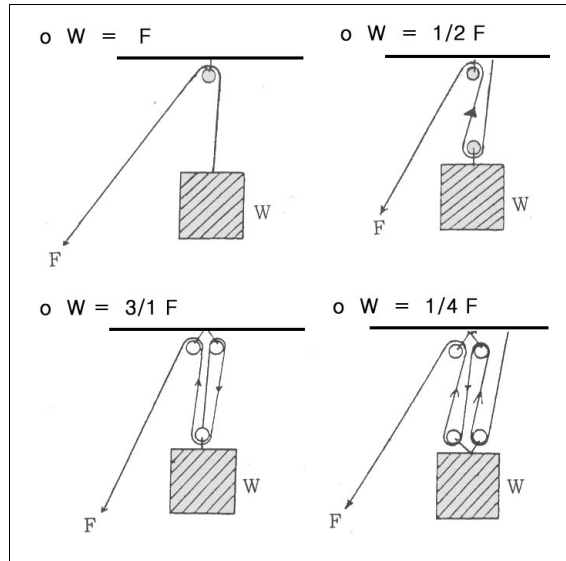
(그림 2-28) 도르래 숫자와 힘의 이득 관계
