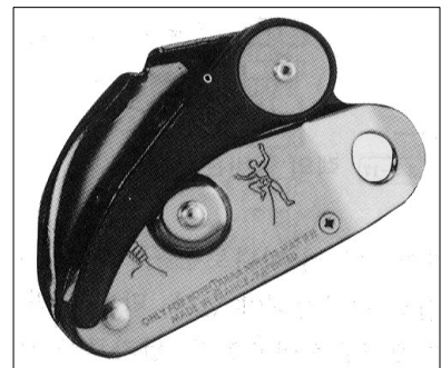
(그림 2-23) 그리그리
