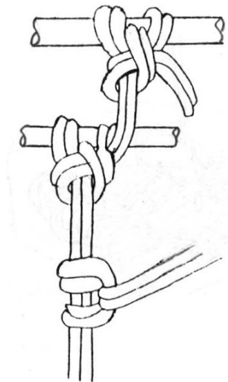
(그림 3-38) 로프 절단이나 지지물의 파손으로 인한 안전사고를 방지하기 위해 로프는 2개소 이상에 결착한다.
