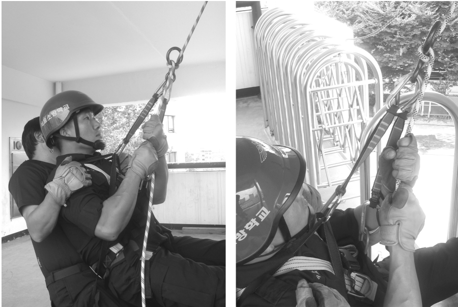
(그림 4-10) 두개의 퀵드로를 이용해서 체중을 분산시킨다.
