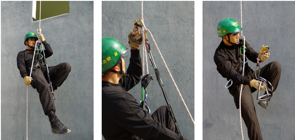
(그림 3-87) 고리를 밟고 몸을 일으켜 세우면서 상승하고 로프를 당겨 올린다. 로프를 쥘마의 카라비나에 넣으면 로프를 당기기 쉽다. 작업이 끝나면 쥘마를 빼고 그리그리를 이용해서 하강한다.
