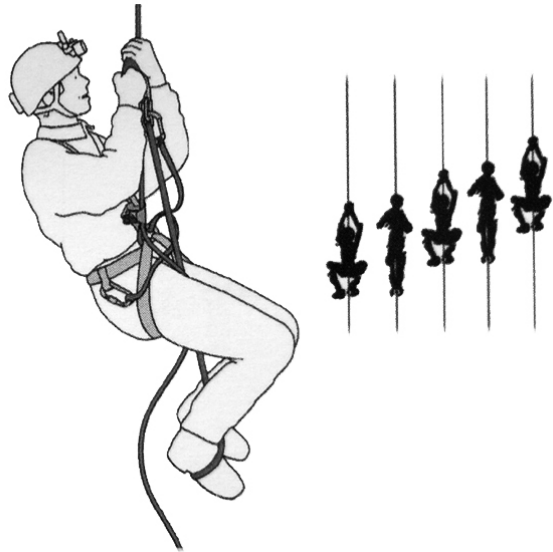
(그림 3-84) 쥘마를 이용한 수직상승 방법
