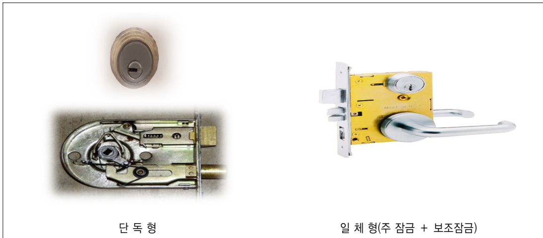
(그림 6-3) 보조 잠금장치의 구조
