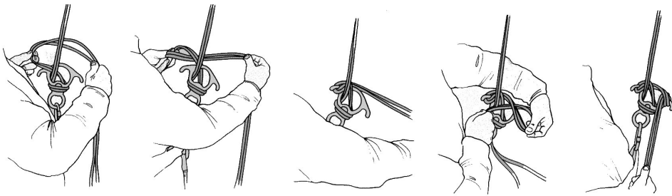
(그림 3-79) 구조용 하강기를 고정하는 방법
