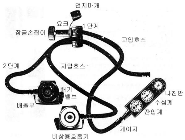
(그림 5-69) 호흡기(Regulator)
