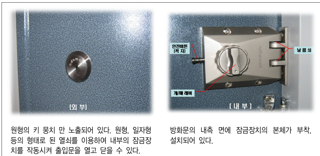
(그림 6-4) 보조 잠금장치
