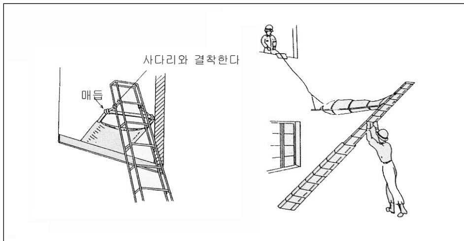
(그림 4-23) 사다리를 이용한 수평구출 방법
