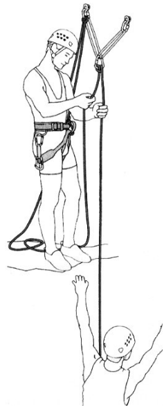
(그림 5-123) 매달아서 내리기
