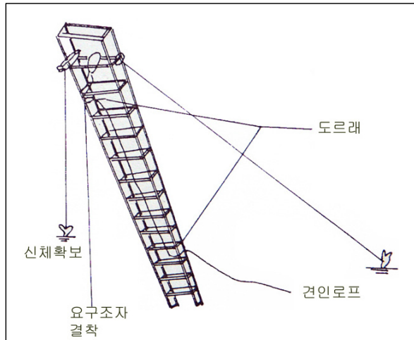
(그림 4-24) 인양구출 로프 설치방법
