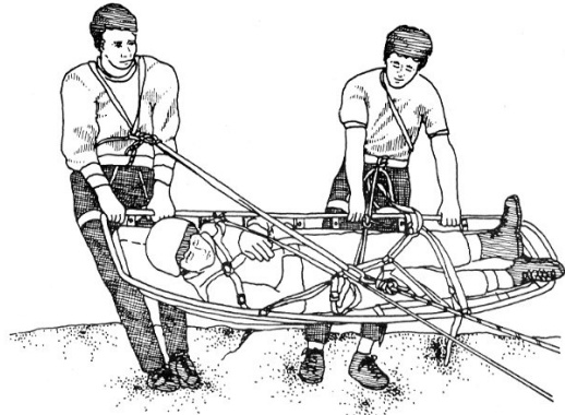
(그림 5-125) 1줄 로프로 하강하기
