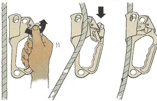
(그림 2-26) 등반기를 로프에 삽입하는 방법
