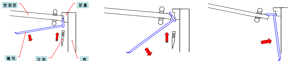
(그림 6-25) 지렛대 활용 작업(4)
