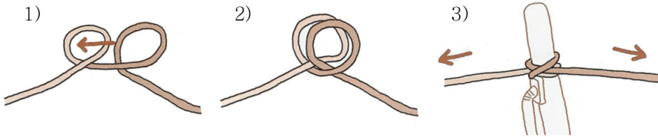
(그림 3-21) 말뚝매기의 다른 방법. 로프 끝을 둥글게 겹쳐서 끼운다.
