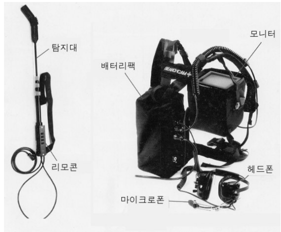
(그림 2-19) 서치캠 (ST-5B)
