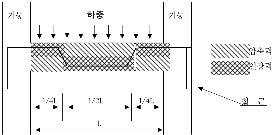
(그림 5-81) 보의 응력 분포
